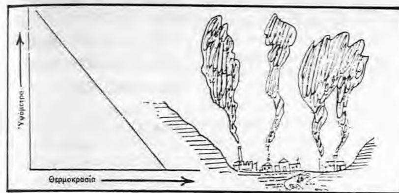
Παράσταση 1. Ουδεμία θερμοκρασιακή αναστροφή
