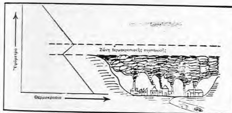
Παράσταση 2. Θερμοκρασιακή αναστροφή
