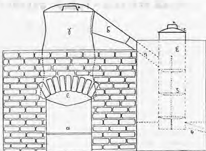
ΣΧΕΔΙΟ ΑΠΟΣΤΑΚΤΗΡΑ ΣΤΕΜΦΥΛΕΝ:
