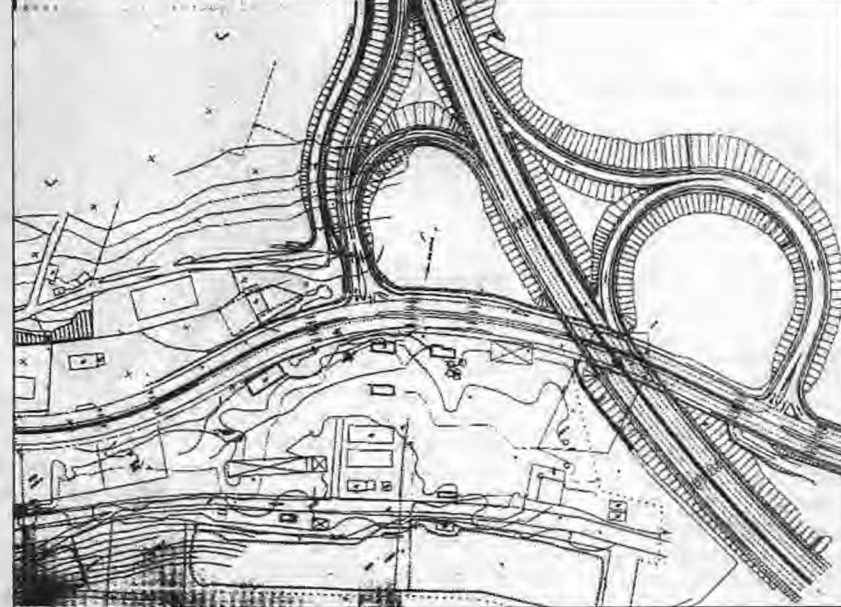
Βάση αυτού του σχεδιαγράμματος θα δουλέψουν οι μηχανικοί για την κατασκευή του κόμβου στη νέα εθνική οδό στη Βέροια.
