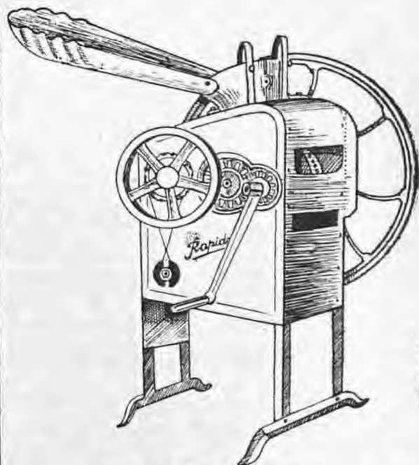
ΕΚΚΟΚΙΣΤΙΚΗ ΜΕ ΔΥΟ ΣΤΟΜΙΑ
