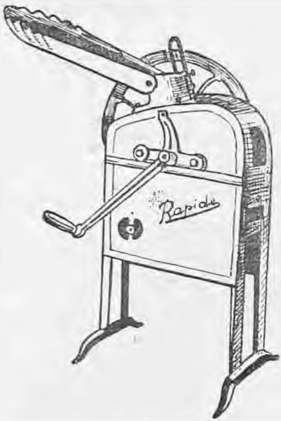
ΕΚΚΟΚΙΣΤΙΚΗ ΜΕ ΕΝΑ ΣΤΟΜΙΟΝ με Ρουλεμάν και άνευ Ρουλεμάν Βάρος μόνον 60 χιλιόγραμμα Παραγωγή 250 άκάδες καθ' ώραν
