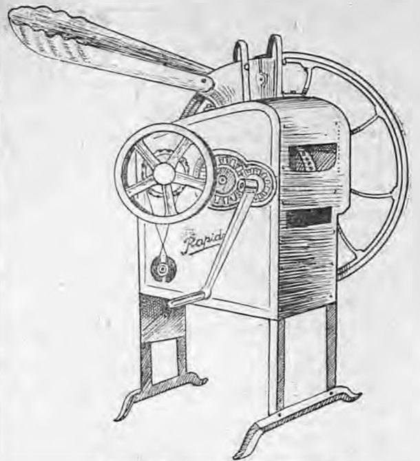
ΕΚΚΟΚΙΣΤΙΚΗ ΜΕ ΔΥΟ ΣΤΟΜΙΑ με Ρουλεμάν και άνευ Ρουλεμάν Χειροκίνητη Μηχανοκίνητη μεγάλης απόδοσεως Βάρος 105 χιλιόγραμμα
