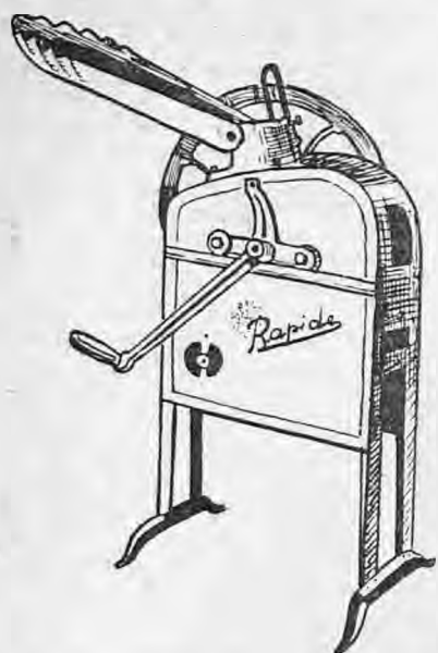
ΕΚΚΟΚΙΣΤΙΚΗ ΜΕ ΕΝΑ ΣΤΟΜΙΟΝ με Ρουλεμάν καὶ ἄνευ Ρουλεμάν Βάρος μόνον 60 χιλιόγραμμα Παραγωγή 250 ἐκάδες καθ' ὥραν
