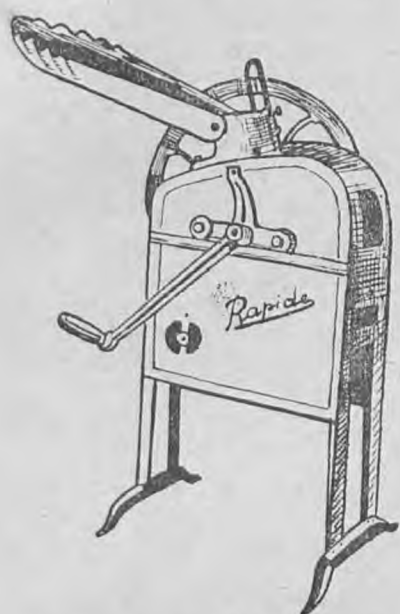
ΕΚΚΟΚΙΣΤΙΚΗ ΜΕ ΕΝΑ ΣΤΟΜΙΟΝ Βάρος μόνον 62 χιλιόγραμμα Παραγωγή 250 όκάδες καθ' ώραν
