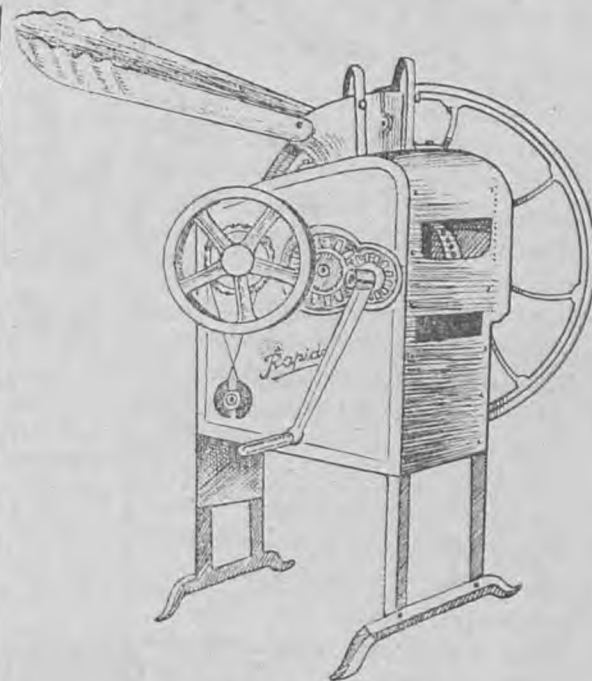
ΕΚΚΟΚΙΣΤΙΚΗ ΜΕ ΔΥΟ ΣΤΟΜΙΑ Χειροκίνητη Μηχανοκίνητη μεγάλης απόδοσης Βάρος 105 χιλιόγραμμα
