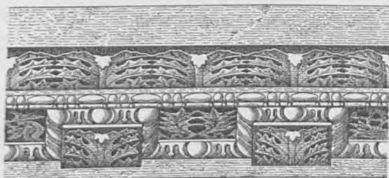
Σχ. 334. Πρόσῃς τῆς αὐτῆς κορωνίδος. Κλίμαξ = \frac{1}{30} .
