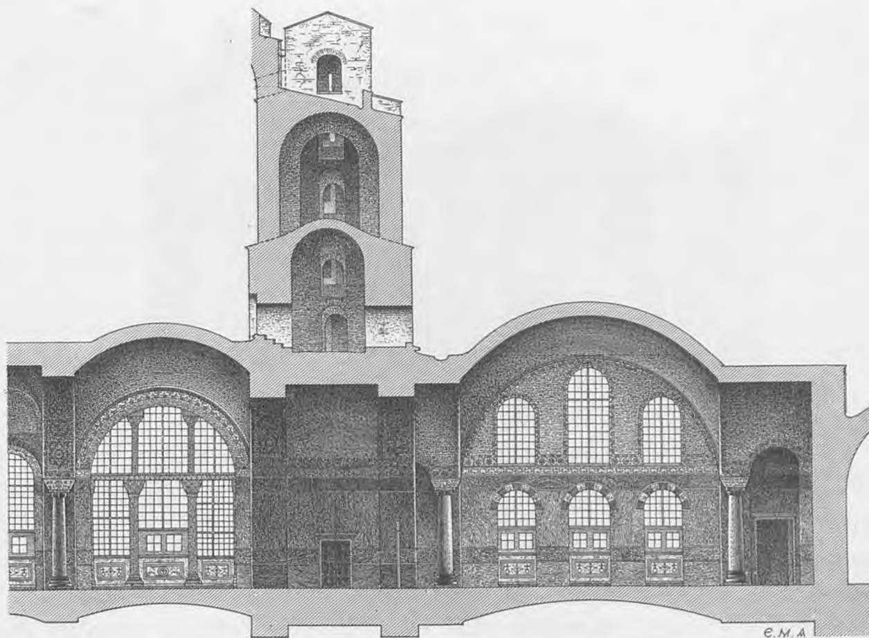
Σχ. 343. Ἡ κατὰ τὸν μείζονα ἀξονα τομὴ τοῦ νοτιοδυτικοῦ τῶν Ὑπερώων διαμερίσματος. Κλίμαξ = \frac{1}{80} .
