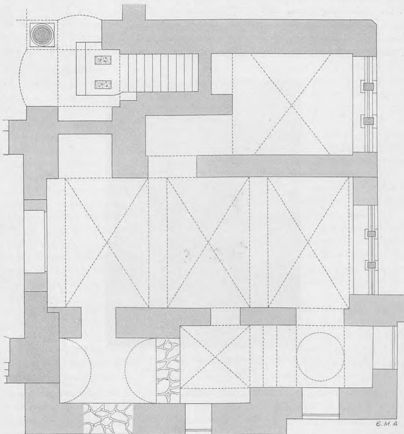
Σχ. 367. Σχεδιάγραμμα τῶν πρὸς νότον τοῦ δυτικοῦ Ὑπερώφου ἐξαρτήσεων. Κλίμαξ = \frac{1}{100} .
