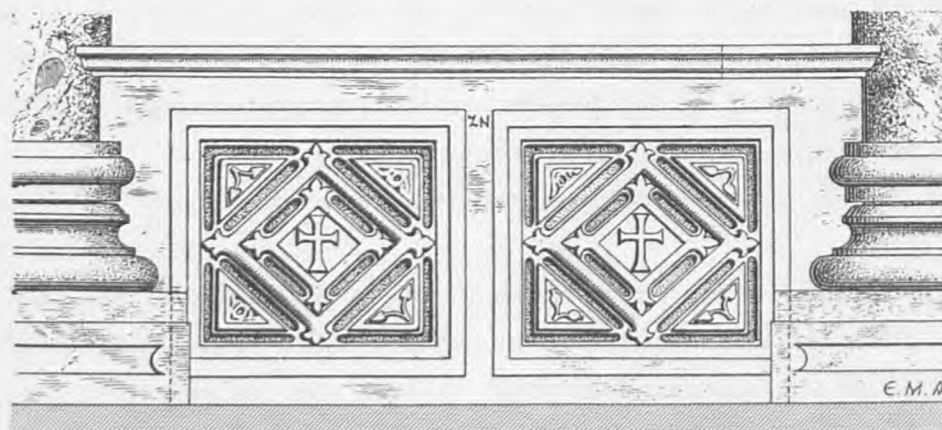
Σχ. 332. Ἡ πρὸς τὸν Ναὸν θέα τοῦ περιφράγματος. Κλίμαξ = \frac{1}{25} .
