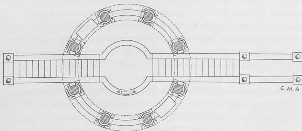
Σχ. 242. Ἀποκατάστασις τοῦ διαγράμματος τοῦ δευτέρου τῆς Ἀγίας Σοφίας Ἀμβωνος. Κλίμαξ = \frac{1}{125} .
