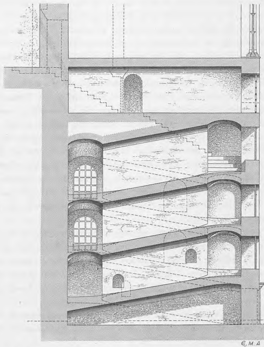
Σχ. 324. Ἡ κατὰ μέσον τῶν ἐσπερίων διαδρόμων παραπλήσια κατακόρυφος τομὴ τοῦ μεσημβρινοδυτικοῦ Λαβυρίνθου. Κλίμαξ = \frac{1}{125} .
