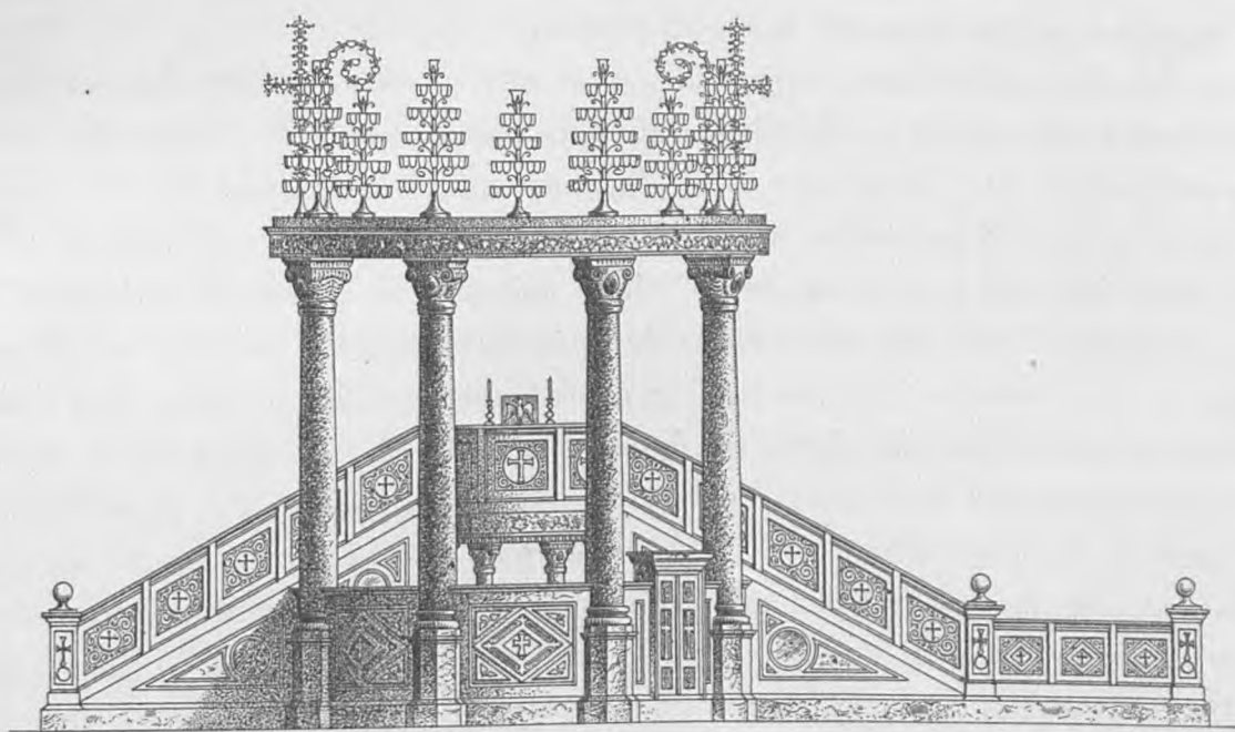
Σχ. 243. Ἀποκατάστασις τῆς μεσημβρινῆς προσόψεως τοῦ αὐτοῦ. Κλίμαξ = \frac{1}{125} .
