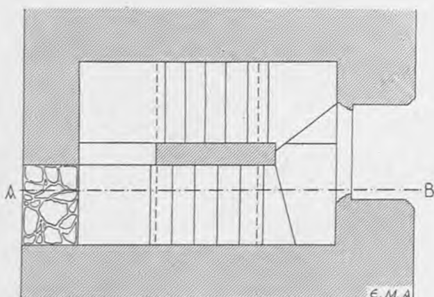
Σχ. 321. Τὸ πρὸς τὸ Ὑπερῶν διάγραμμα τῆς ἐν τῷ μεσημβριοανατολικῷ παραπηρσίῳ ἀνόδου. Κλίμαξ=7 π .
