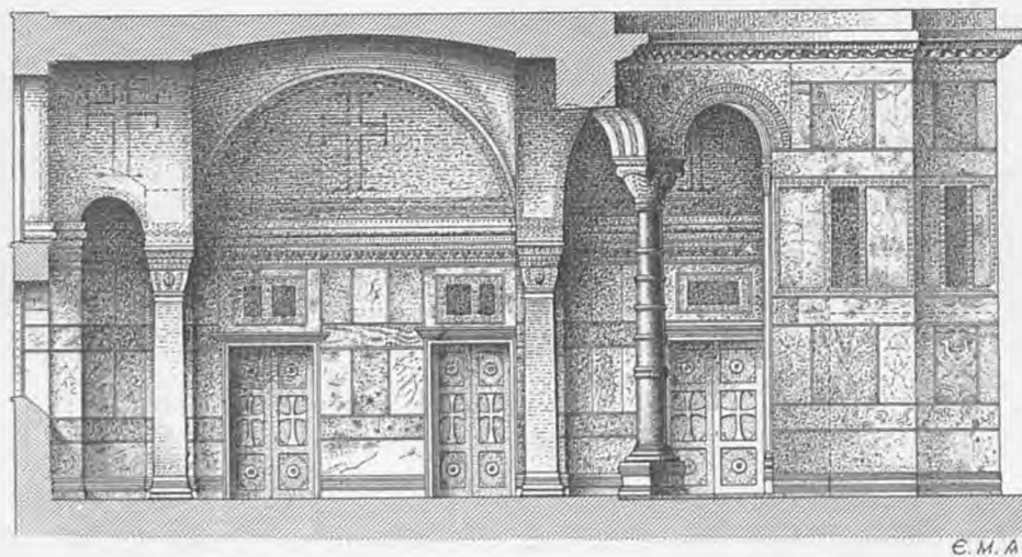
Σχ. 270. Ἡ κατὰ τὸν ἐλάσσονα ἄξονα τομὴ τῆς νοτιοδυτικῆς Στοᾶς. Θέα πρὸς δυσμὰς. Κλίμαξ = \frac{1}{3} \frac{1}{8} .
