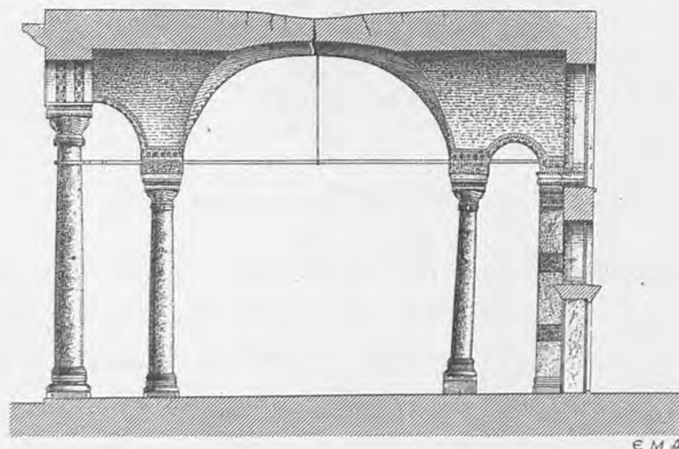
Σχ. 281. Τὸ ἐν τῇ νοτίᾳ Στοᾷ ἀποτέλεσμα τῶν σεισμῶν. Κλίμαξ = \frac{1}{60} .
