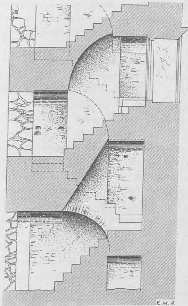
Σχ. 323. Ἡ κατὰ τὴν γραμμὴν ΑΒ τῶν προηγουμένων δύο σχημάτων κατακόρυφος τομὴ τῆς νοτιοανατολικῆς ἀνόδου. Κλίμαξ— \frac{1}{2} σ.
