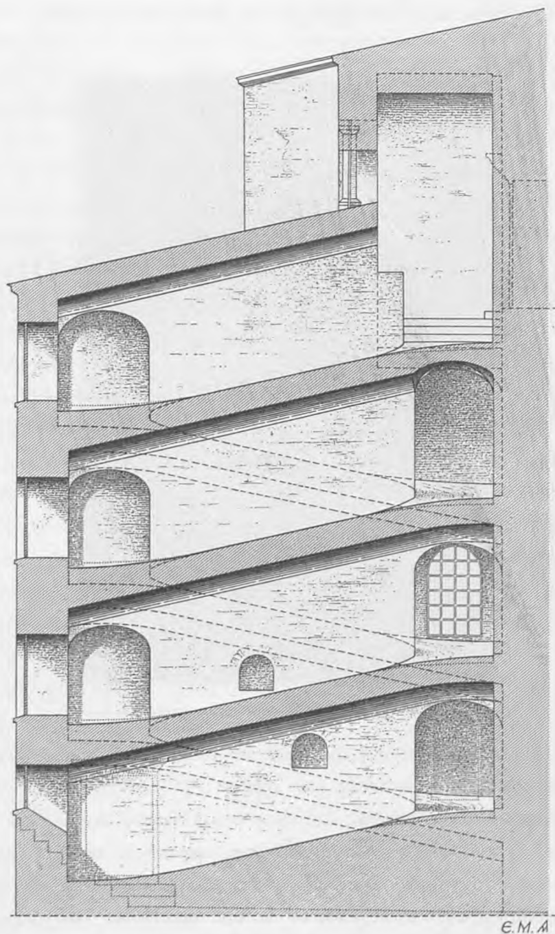
Σχ. 326. Ἡ κατὰ μέσον τῶν ἐσπερίων διαδρόμων παραπλησία κατακόρυφος τομὴ τοῦ βορειοδυτικοῦ Λαβυρίνθου. Κλίμαξ = 1\frac{1}{2} .
