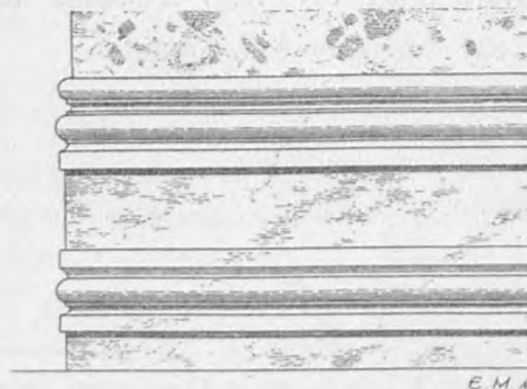
Σχ. 202. Βάσις τῆς τοῦ Ναοῦ ὀρθομαρμαρώσεως. Κλίμαξ = \frac{1}{2}\delta .
