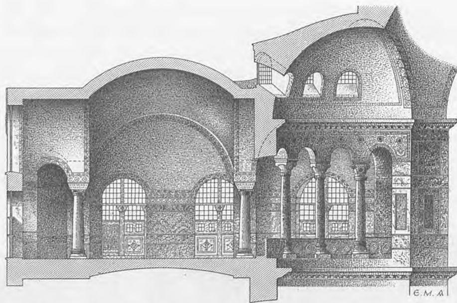
Σχ. 344. Τομή κατὰ τὸν ἐλάσσονα ἄξονα τοῦ νοτιοδυτικοῦ Ὑπερφῶν. Κλίμαξ = \frac{1}{250} .
