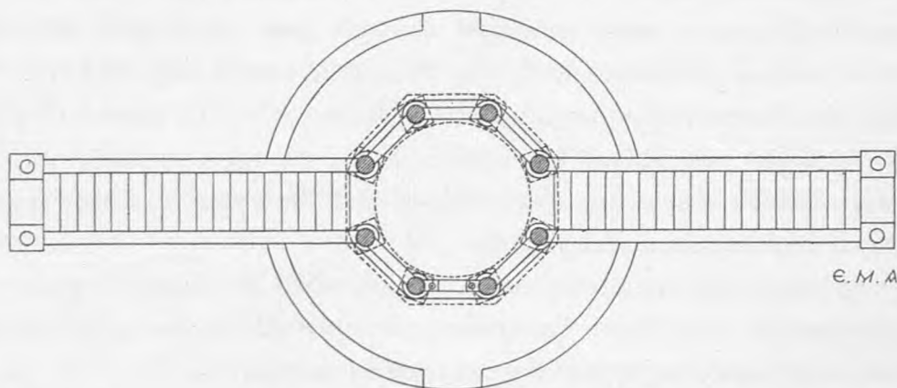
Σχ. 244. Ἀποκατάστασις διαγράμματος τοῦ τελευταίου τῆς Ἀγίας Σοφίας ἄμβωνος. Κλίμαξ=1½.
