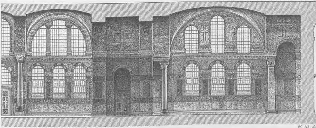
Σχ. 269. Ἡ κατὰ τὸν μείζονα ἄξονα τομὴ τῆς νοτιοδυτικῆς Στοᾶς.
