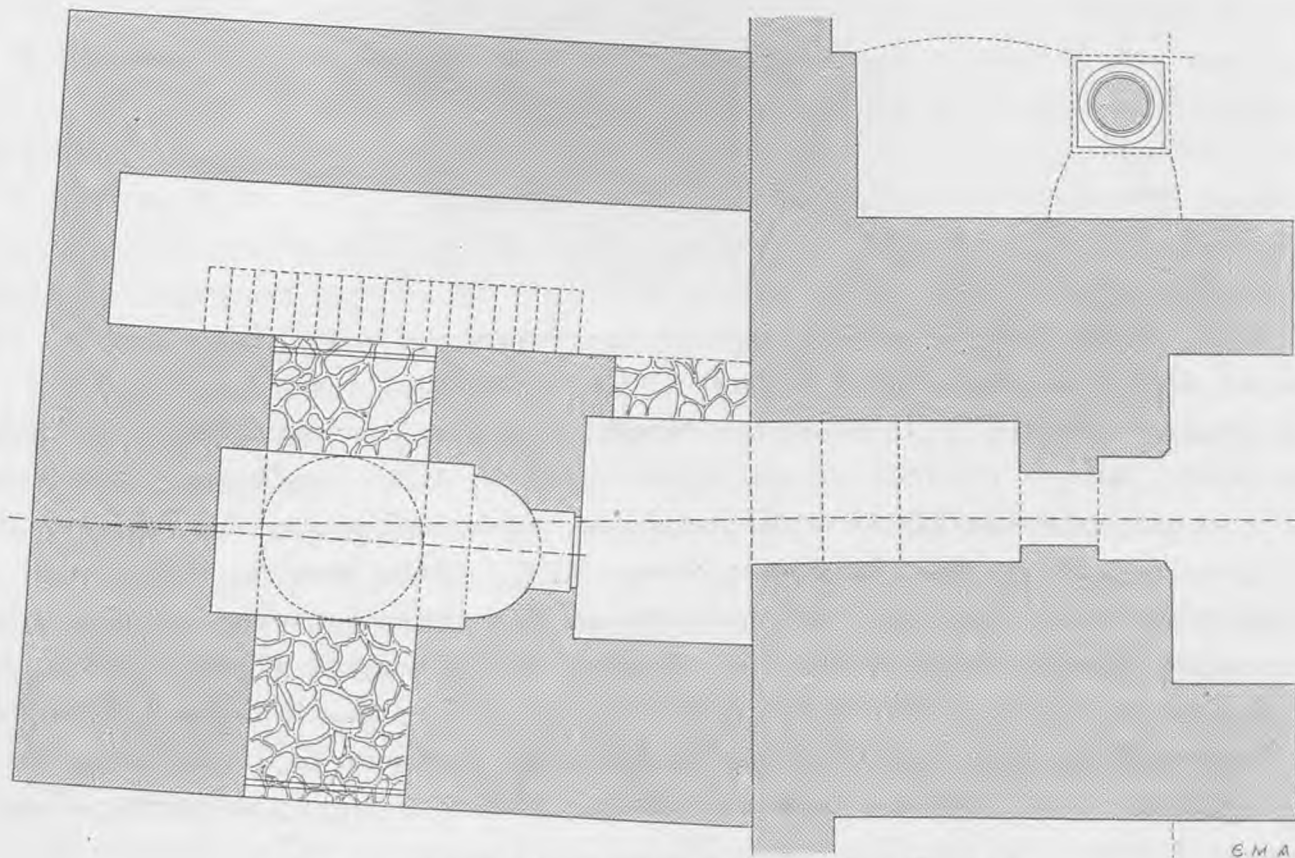
Σχ. 397. Διάγραμμα τοῦ μεσημβρινοδυτικοῦ παρεκκλησίου. Κλίμαξ=1/100.
