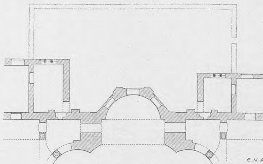
Σχ. 262. Ἀποκατάστασις τῆς πιθανῆς ἀρχικῆς διατάξεως τοῦ παρὰ τὸ Βῆμα τοίχου. Κλίμαξ = \frac{1}{500} .
