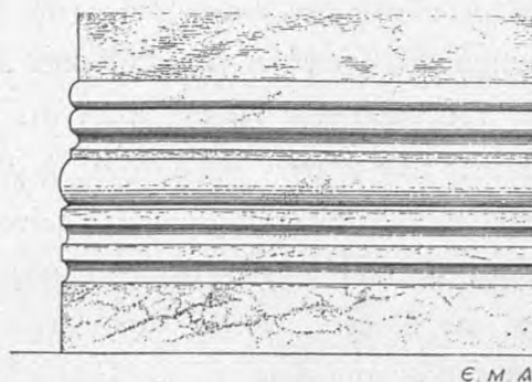
Σχ. 272. Βάσις τῆς τῶν Στοῶν ὀρθομαρμαρώσεως. Κλίμαξ = 1/10.
