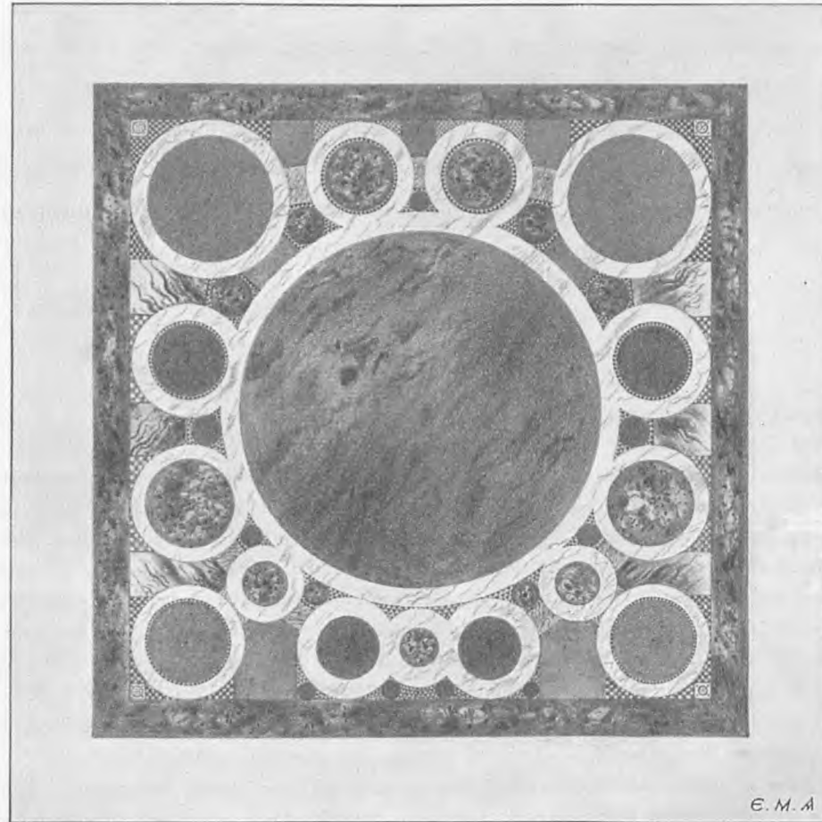
Σχ. 237. Παραπλησία θέα τοῦ ἐν τῷ Ναῷ Ὀμφαλίου. Κλίμαξ = \frac{1}{80} .
