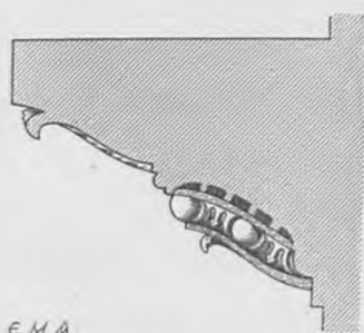
Σχ. 333. Κατατομή τῆς τοῦ Ὑπερώου κορωνίδος. Κλίμαξ = \frac{1}{30} .
