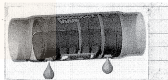
Εικ. 2 Στακτοφόρος σωλήνας Hydro P.C
