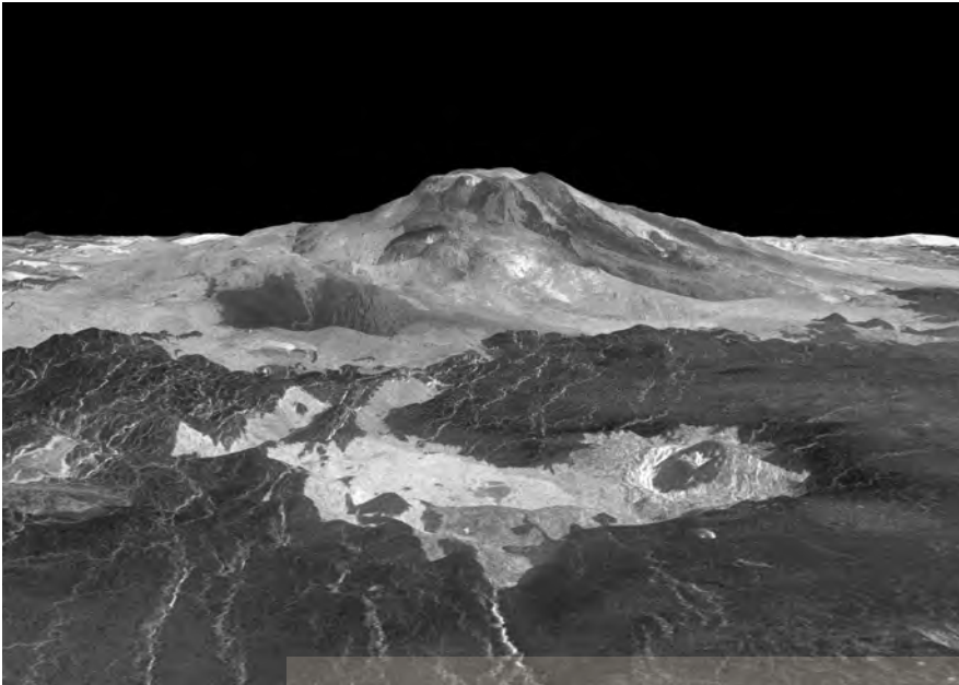
Η επιφάνεια του πλανήτη Αφροδίτη και το ηφαίστειο Maat Mons
