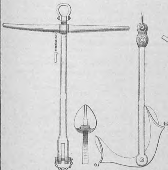
3. Ὀνυχάρθρωτος ἄγκυρα
