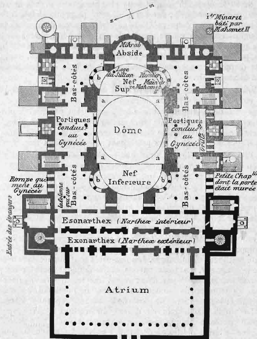
Plan de Sainte Sophie d'après Fossati et Batissier.
