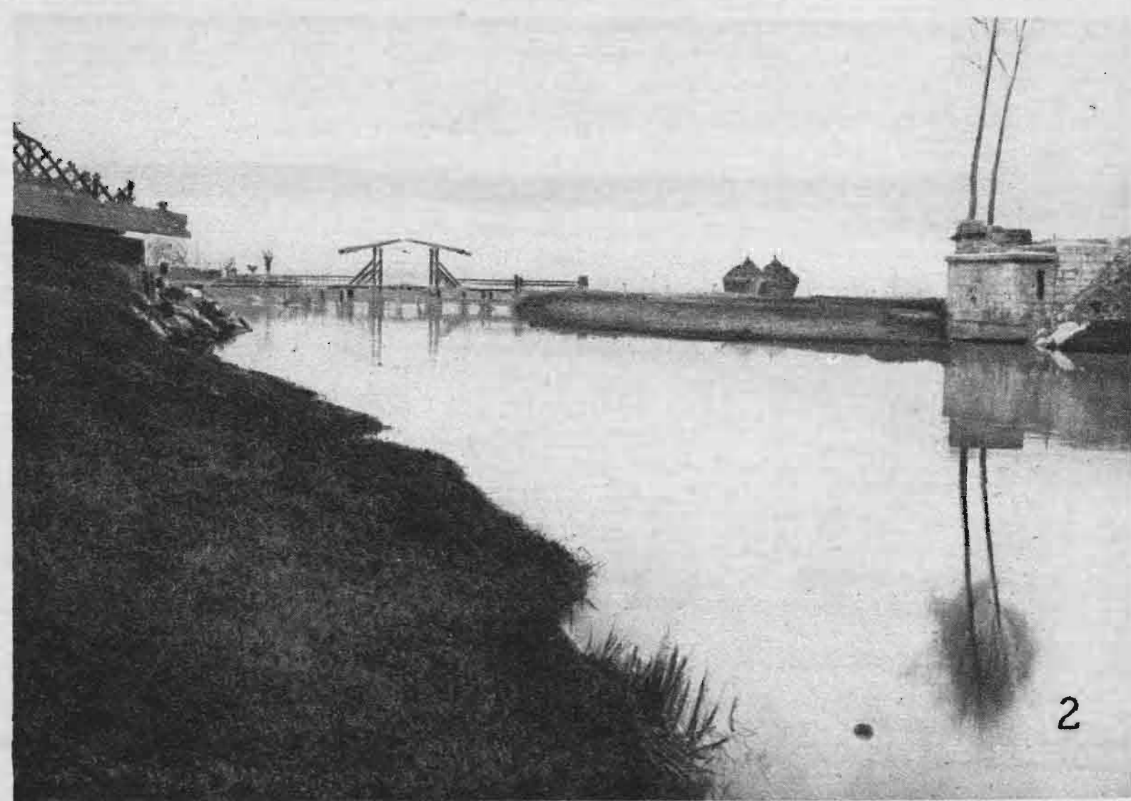
Wiederaufbau einer von den Bel- giern zerstörten Brücke durch deutsche Pioniere.
