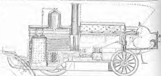
2. Έσωτερική διάταξις ιδιοστραμίδης.
