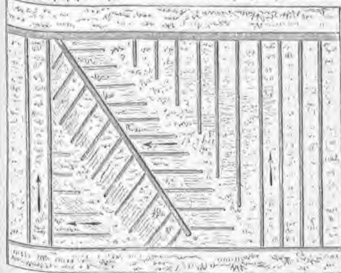
15. Συνθετον αποστραγγιστικόν σύστημα.
