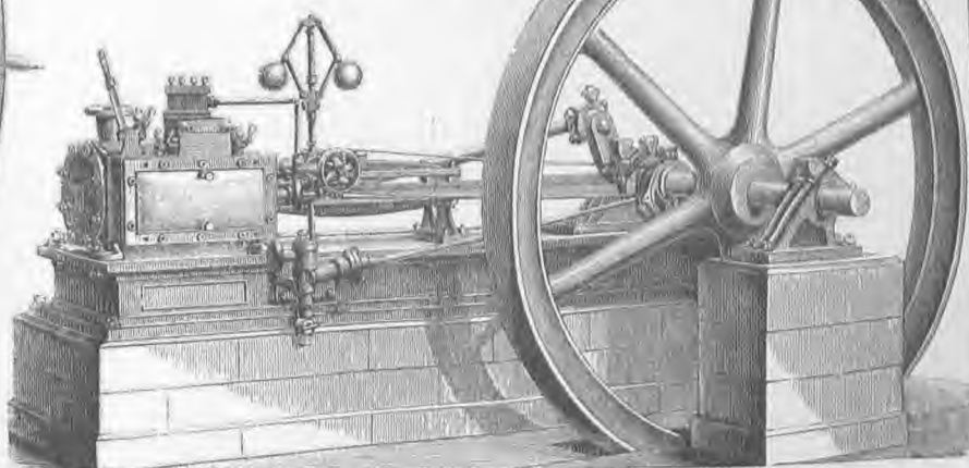
10. Οριζόντιος ατμομηχανή.
