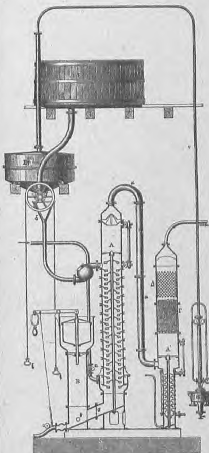
3. Συνεχῆς ἀποστακτικὴ συσκευή τοῦ Ilges.
