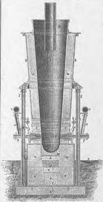
1. Κάμινος του Πίλτζη.
