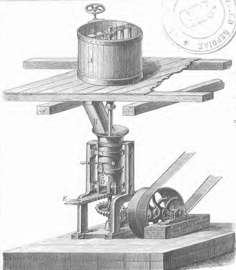
2. Ζυμωτική μηχανή του Βορβέκερ.
