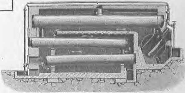
12. Διάταξις τῆς θερμάνσεως τοῦ Ten-Brink λέβητος.
