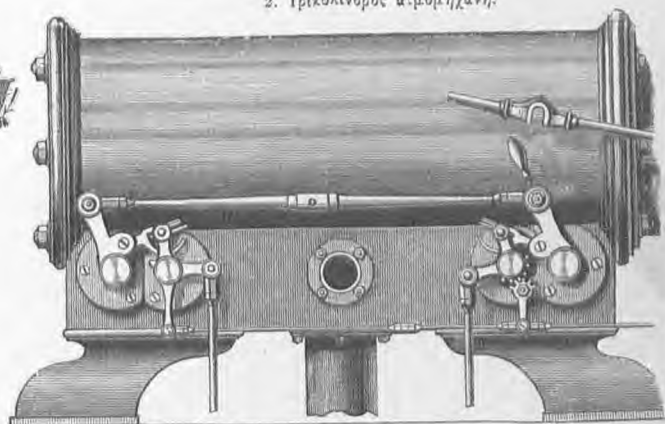
4. Ἀτμομηχανὴ Κόρλις συνστ. Θύλλοι.
