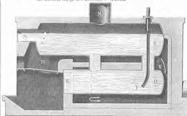
1. Συνήθης αεριολέβης μετά προθερμαστήρος.
