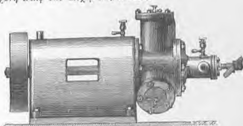
2. Τρικύλινδρος ἀτμομηχανή.
