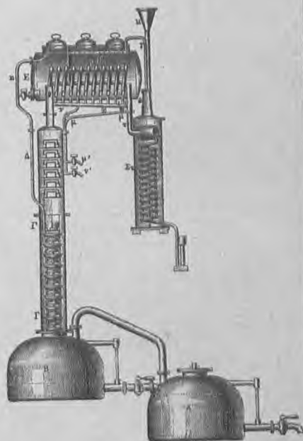
2. Ἀποστακτικὴ συσκευή τῶν Cellier-Blumenthal-Derosue
