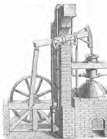
8. Ατμομηχανή Newcomen.
