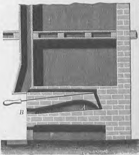
4. Κλίβανος πυροόμενος διά ξύλων.
