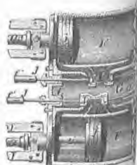
4. Έσωτερική διάταξις κυλίνδρων ατμομάζης.
