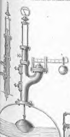
8. Μαγνητικός υδραυλικός.
