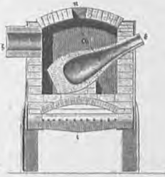
6. Τομή προσθία.
