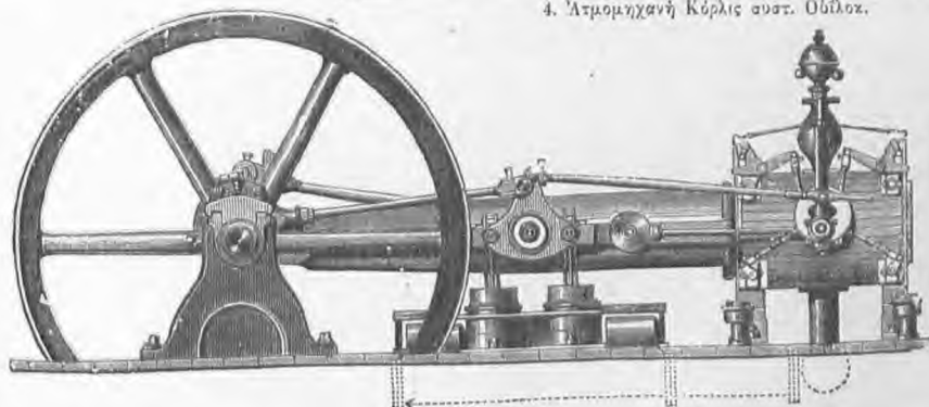
5. Ἀτμομηχανὴ Κόρλις.
