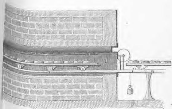
Κλίβανος πυροόμενος δι' ύδατος.
