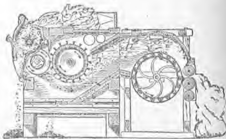
(Σχ. 4) Κόβτης τοῦ ἐκκοκιστικῆς Emery μετὰ συμπνευστήρι.
