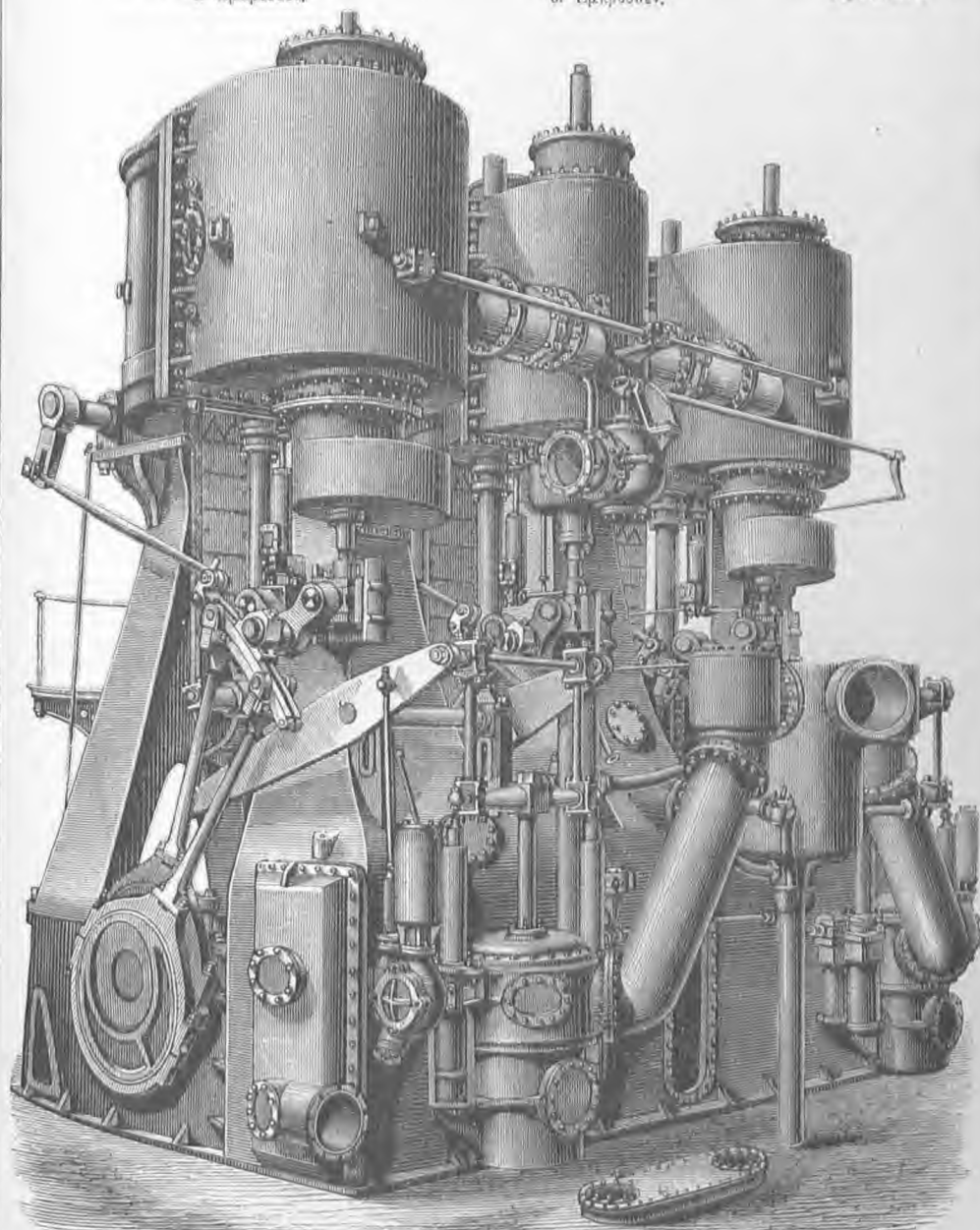
1. Τρικύλινδρος μηχανή ατμοπλοίου συστήματος Compound (πλάγια όψις).
