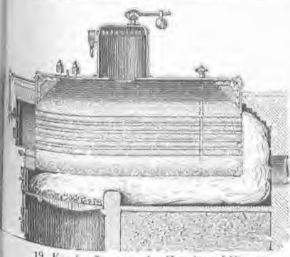
19. Κατά μέγεθος τομή ατμοφόρου λέβητος.
