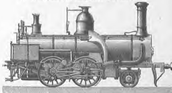
7. Ὀρειβατικὴ ατμόμαζα.
