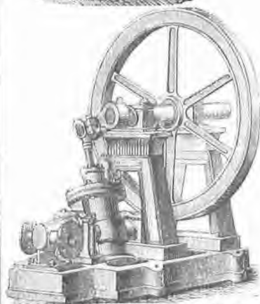
7. Περαινεύουσα ατμομηχανή του Hick.
