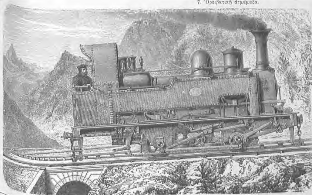
12. Ὀρειβατικὴ ατμόμαζα συστ. Φέλς.
