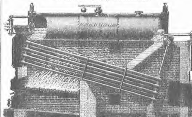
11. Αύλωτος λέβης υπό Babcock & Wilcox.
