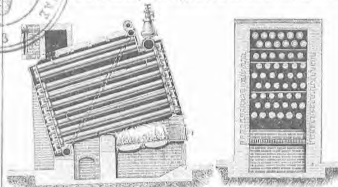
14. 15. Αύλωτος λέβης υπό Rootsocher.
