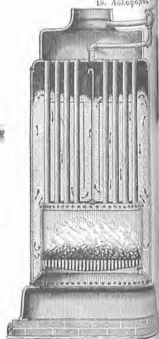
9. Όρθιος αύλωτος λέβης.
