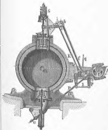
3. Ἀτμομηχανὴ Σουλτσερ.
