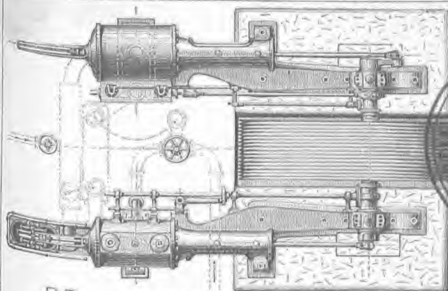
1. Σύστημα ατμομηχανή Κόλμαν.
