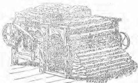
(Σχ. 3) Ἀπλῆ πλῆρᾳ ἐκκοκιστικῆς Emery ἐν ἰσχυρῇ μετὰ συμπνευστήρι.
