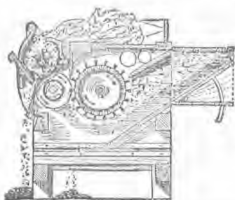
(Σχ. 1) Κόβτης τοῦ ἀπλῆς ἐκκοκιστικῆς Emery
