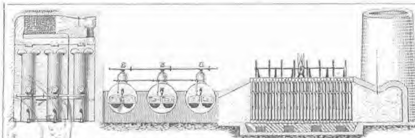
17. Διάταξις συσκευής προς θέρμανσιν του ύδατος των λεβήτων (σίκανόμας).
