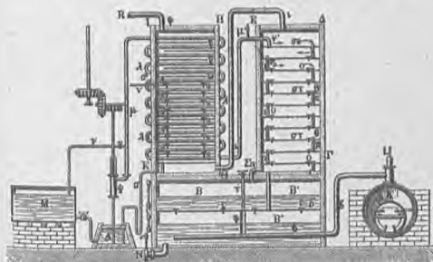
Ἀποστακτικὴ συσκευή του Coffey.
