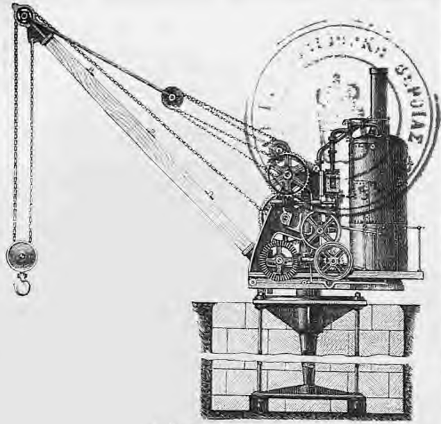
5. Γέρανος ατμοκίνητος.
