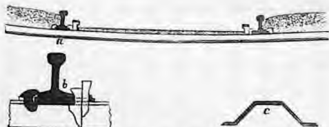
20. a. b. c. Σύστημα σιδηρῶν ἐγκαρσίων στρωτήρων.
