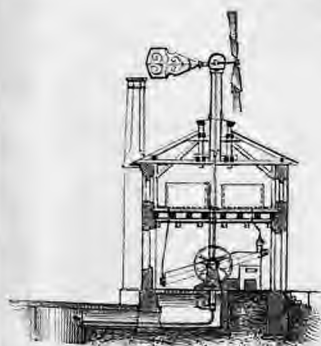
5. "Γόρτυμα δι' άνεμομόλου.
