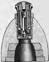
5. Ποροσωλήν κρουσιφόρος.
