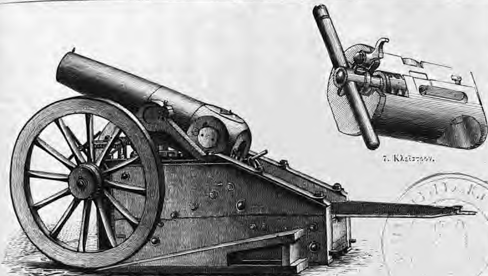
1. Όλμος των 21 έμ.
