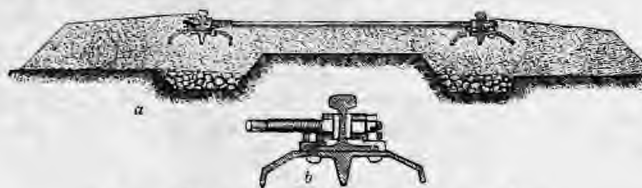
4. α. β. Σύστημα Hill τών κατά μήκος στρωτήρων.
