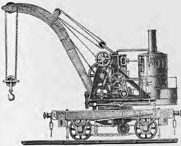
6. Γέρανος εν ατμομάτῃ.
