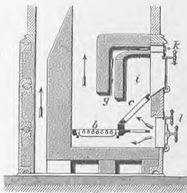
6. Πηλίνη θερμ. μετ' ἀκάπνου καύσεως.
