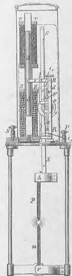
8. Ἡλεκτρ. λύχνος Σμιενς-Αλσκε.
