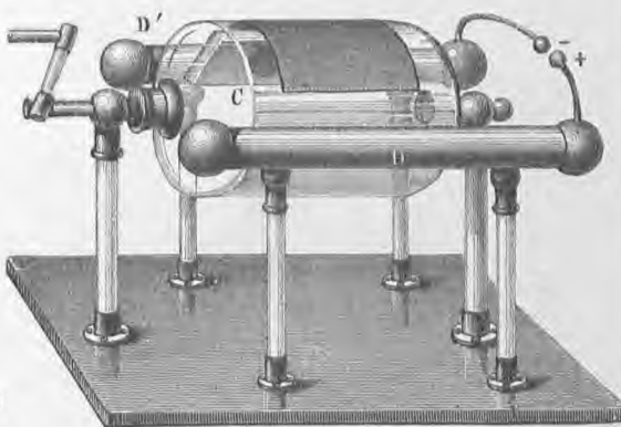
9. Κυλινδροφόρος μηχανὴ τοῦ Ναιρν.
