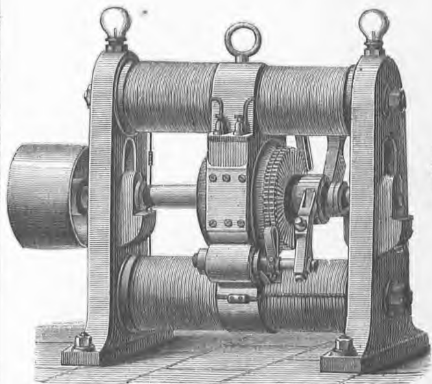
11. Ηλεκτρομηχανή του Γράμμ.
