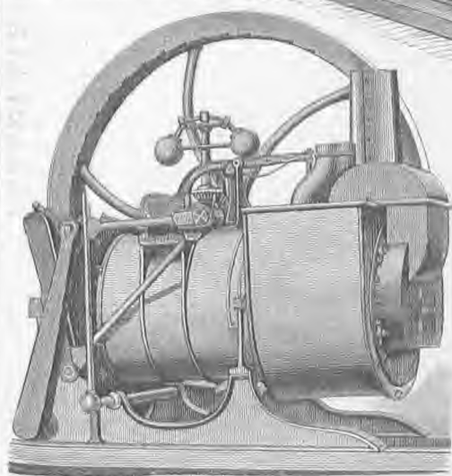
2. Μηχανή του Έρικσον.
