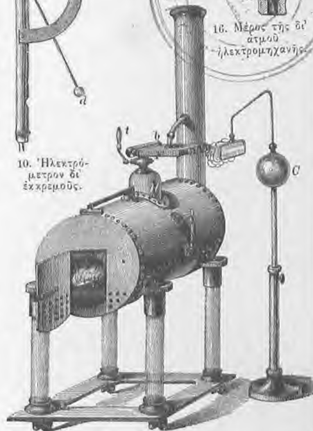
14. 'Ηλεκτρομηχανή δι' ατμού.
