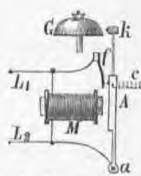
3. Μηχανισμὸς ἡλεκτρικοῦ κώδωνος.
