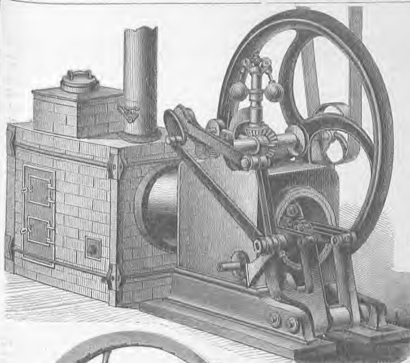
1. Μηχανή του Λίμαν.
