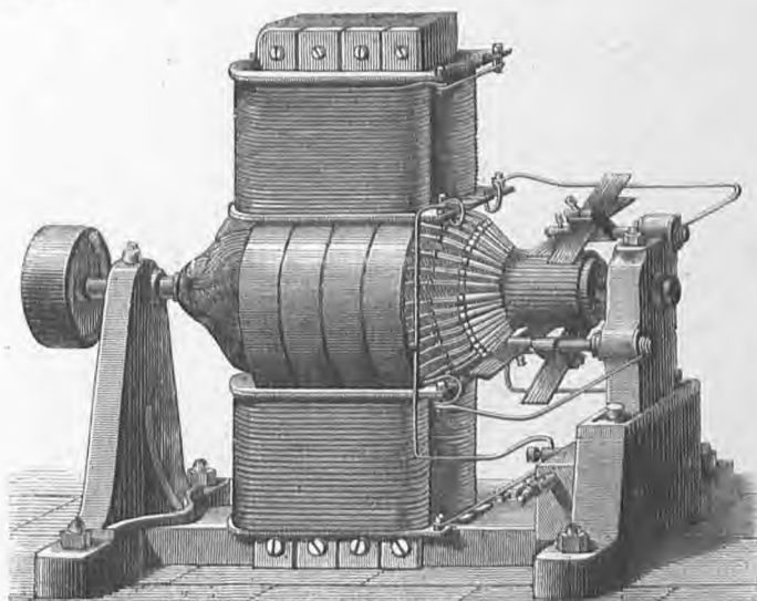
13. Δυναμοηλεκτρική μηχανή Σίμενς-Άλσκι.
