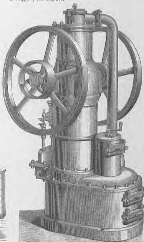
3. Μηχανή του Ου.
