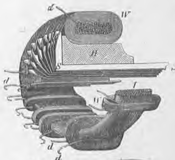
12. Δακτύλιος μηχανής Γράμμ.
