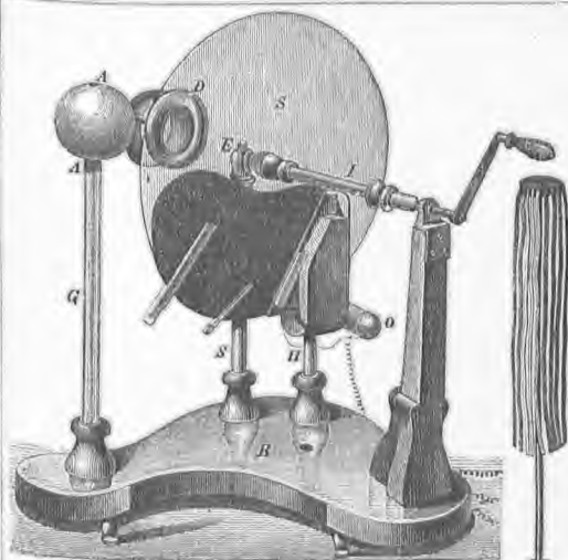
7. Δισκοφόρος ηλεκτρομηχανή.
