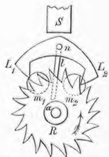
5. Μηχανισμὸς ἡλεκτροκίνητου ὥρολόγιου.
