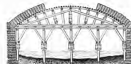
11. Τύπος θόλου λιθίνης γέφυρας.
