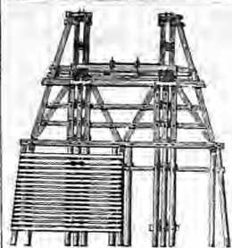
1. Εγκαταστάσι τῆς γέφυρας συστ. Howe.
