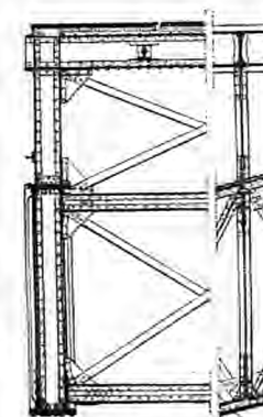
8. Λεπτομέρεια τῆς ἐπὶ τοῦ Ῥήνου γέφυρας.
