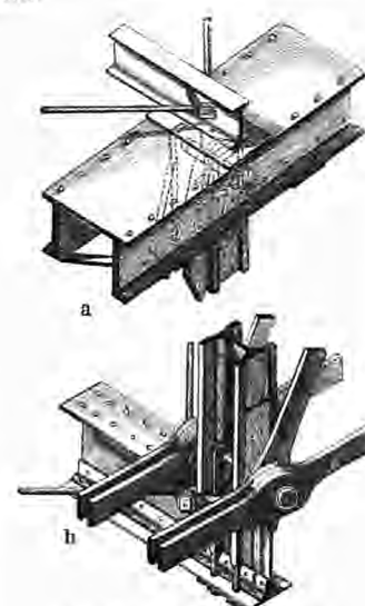
5. Λεπτομέρεια ἀμερικανικῆς δικτυωτῆς γεφύρας.
