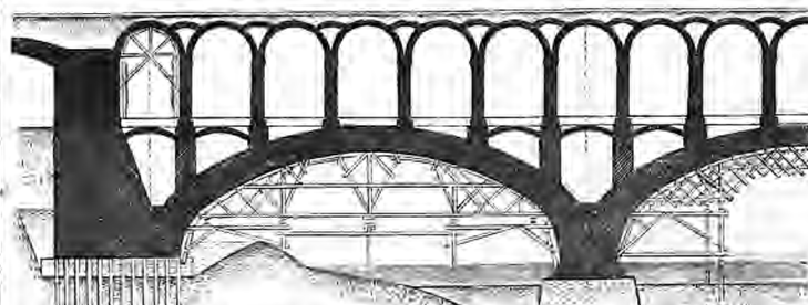
9. Κατὰ μῆκος τομή μιᾶς ἐπὶ τοῦ Σηκουάνης γέφυρας.
