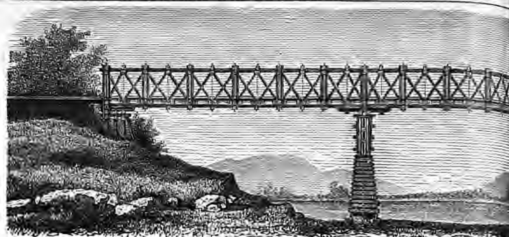
2. Γέφυρα συστ. Howe.
