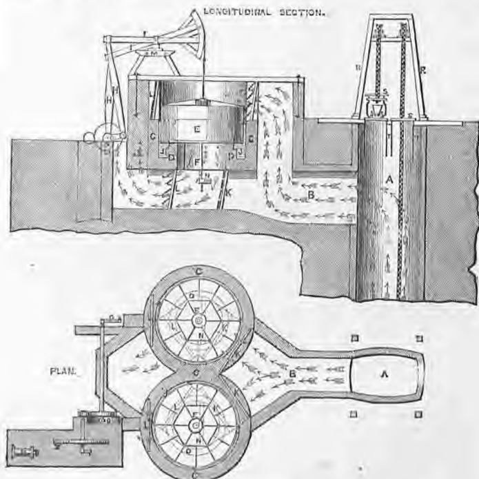
Fig. 43. Strave's Apparatus.
