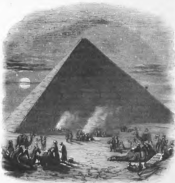
Fig. 17. The Pyramid of Ghizeh.
