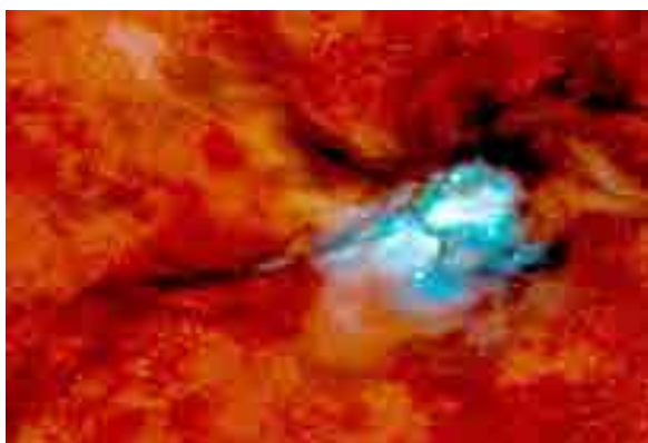
Καλλιτεχνική άποψη της δημιουργίας αστρικού σμήνους από τη σύγκρουση μοριακών νεφών που εικονίζονται ως σκοτεινά νήματα.
