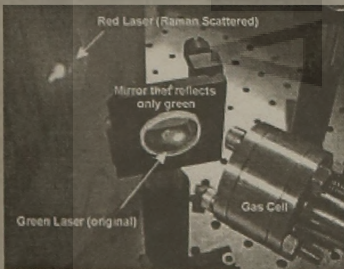
Η πειραματική διάταξη η οποία οδηγεί στο φαινόμενο στην αρχή του οποίου στηρίχθηκε η ανίχνευση
