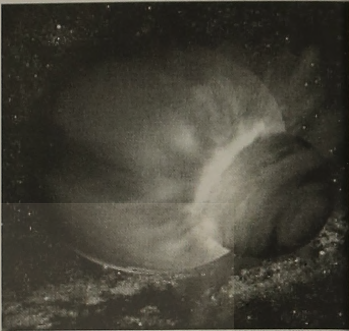
Αναπαράσταση καλλιτεχνική από μια σύγκρουση δυο πρωτοπλανητών, ενός στο μέγεθος του Δία και ενός στο μέγεθος του Ποσειδώνα. (Πηγή: Harvard-Smithsonian CfA)
